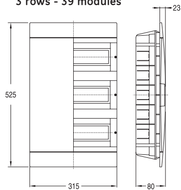
3 rows - 39 modules
