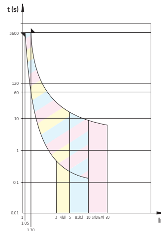
Curve K (EN/IEC 60947-2) versus B, C, D (EN/IEC 60898-1)
