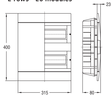
2 rows - 26 modules
